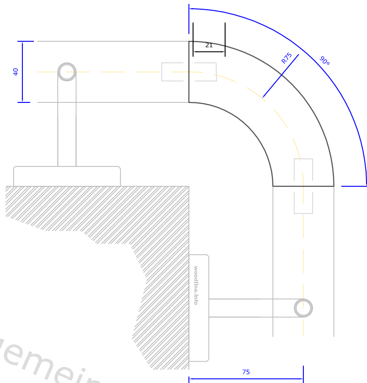
Handlaufbogen 90° für Handlauf Ø 40 mm
