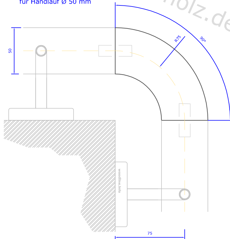
Handlaufbogen 90° für Handlauf Ø 50 mm
