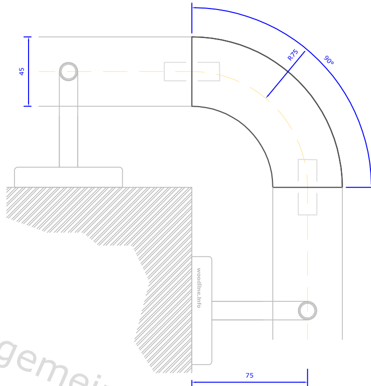
Handlaufbogen 90° für Handlauf Ø 45 mm
