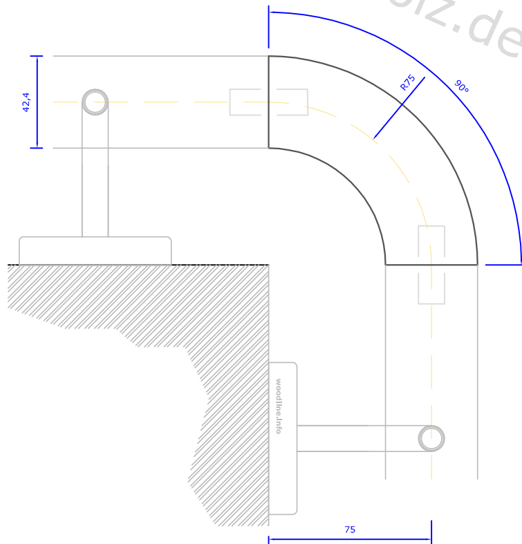
Handlaufbogen 90° für Handlauf Ø 42,4 mm
